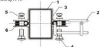
przekrój A-A:
